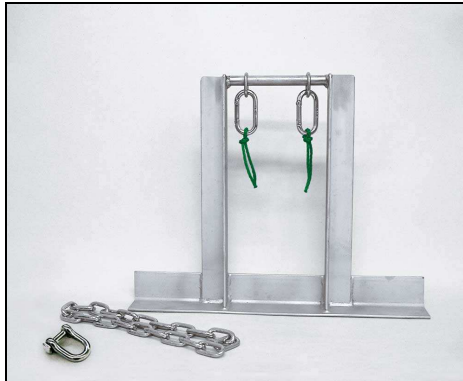
RT-F010996 サッカーゴール固定金具
